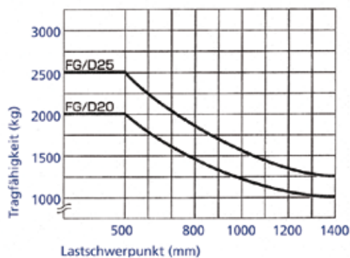
Lasttabelle 2 - 2,5 t
